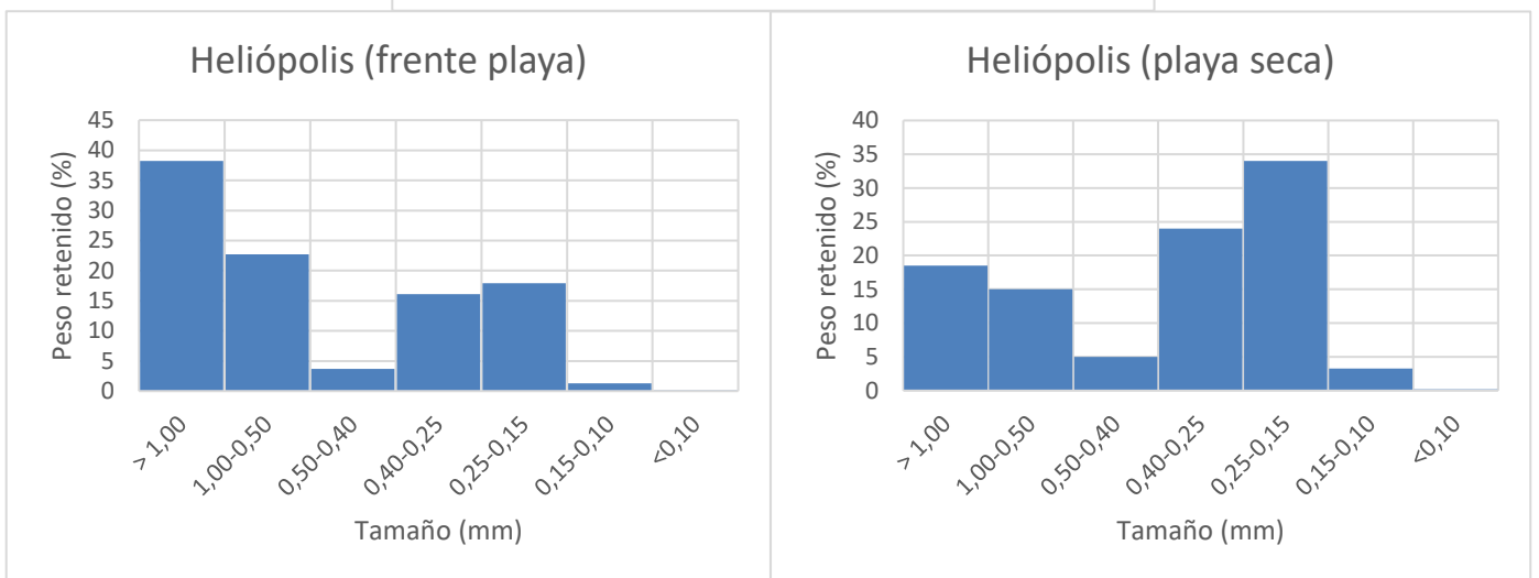
Figura 22. Distribución de tamaños de partícula de las muestras de arena recolectadas en el Torreón y Heliópolis.
