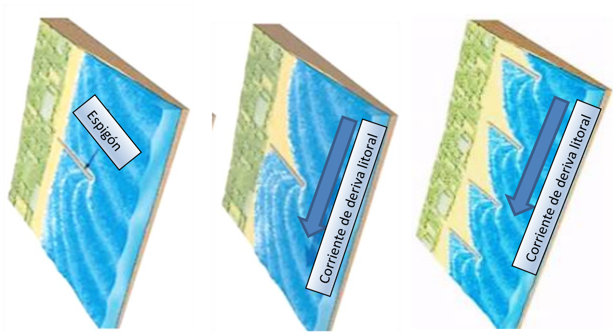
Figura 39. Interrupción de la corriente de deriva consecuencia de la construcción de espigones. Se produce una brusca sedimentación en la zona anterior al obstáculo y una intensa erosión en la posterior.
