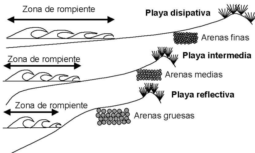
Figura 40. Características de las playas disipativas, intermedias y reflectivas.
